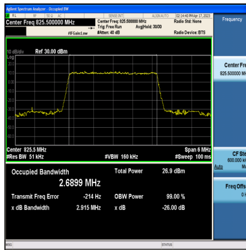
Band5-3MHz-QPSK-20415-15RB#0-2.6899
