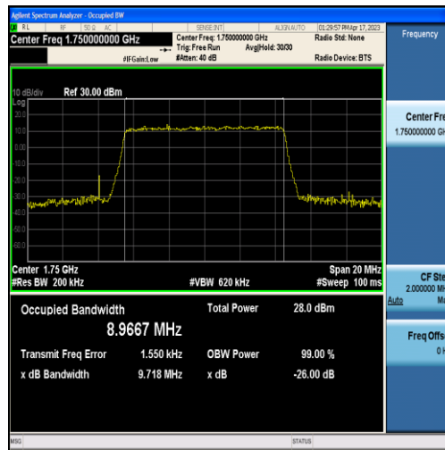
Band4-10MHz-QPSK-20350-50RB#0-8.9667
