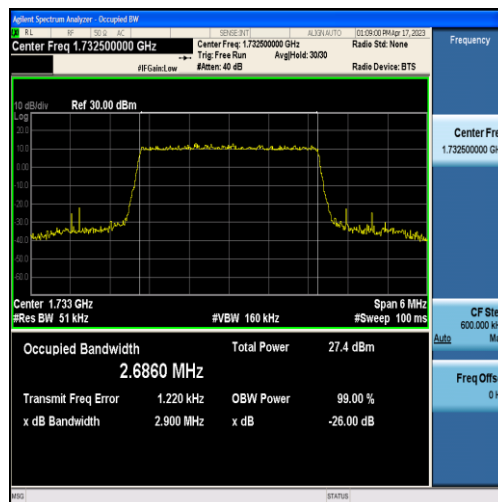
Band4-3MHz-QPSK-20175-15RB#0-2.6860
