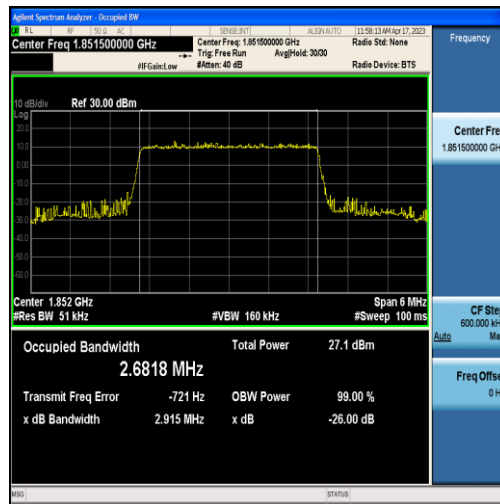
Band2-3MHz-16QAM-18615-15RB#0-2.6818
