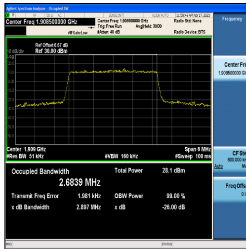
Band2-3MHz-QPSK-19185-15RB#0-2.6839
