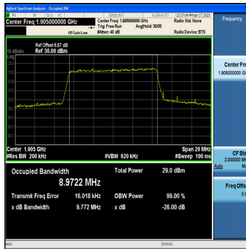
Band2-10MHz-QPSK-19150-50RB#0-8.9722
