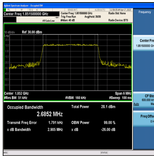
Band2-3MHz-QPSK-18615-15RB#0-2.6852
