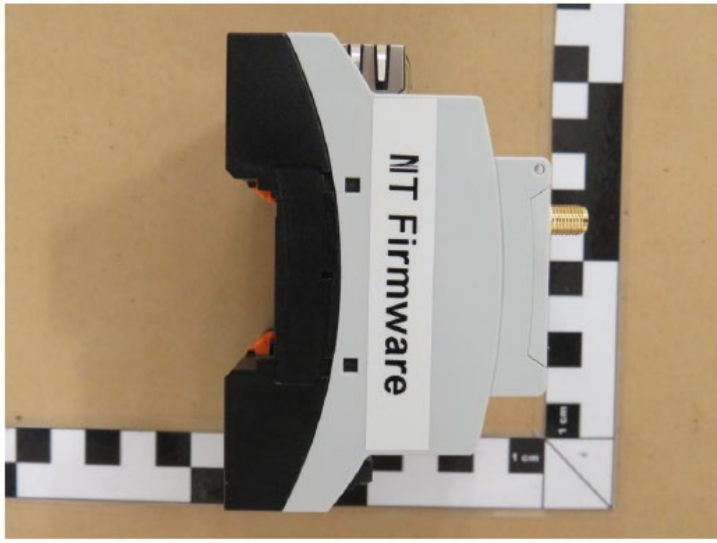
EUT left
