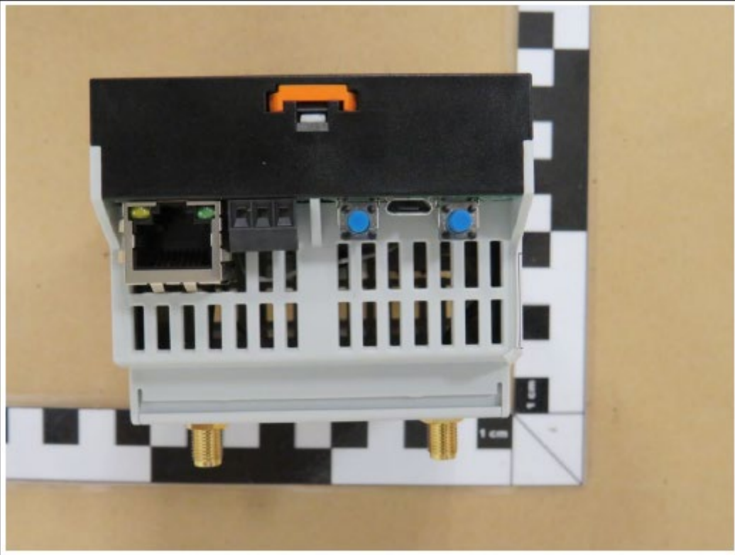
EUT top
