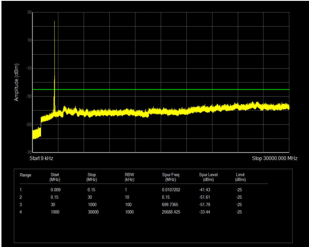
n41 SCS=15kHz DFT_QPSK BW=10MHz Channel=518601 RB=1@51
