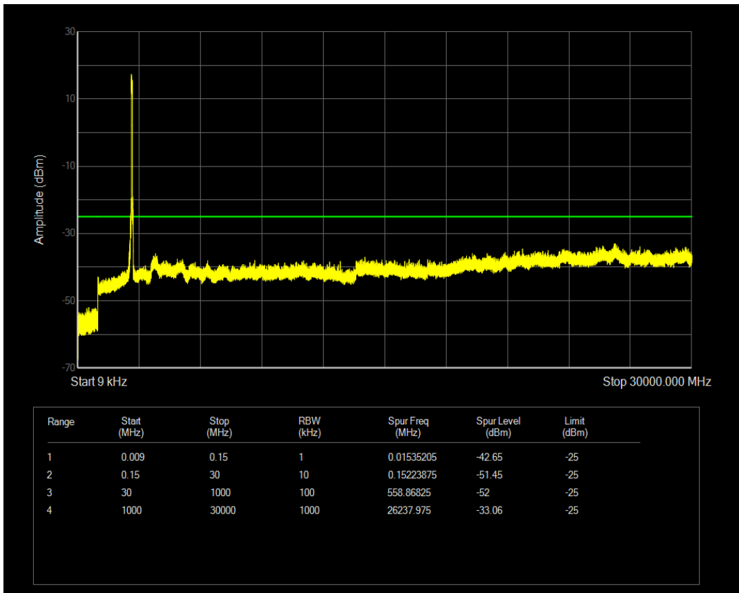
n41 SCS=15kHz DFT_QPSK BW=50MHz Channel=532998 RB=1@0
