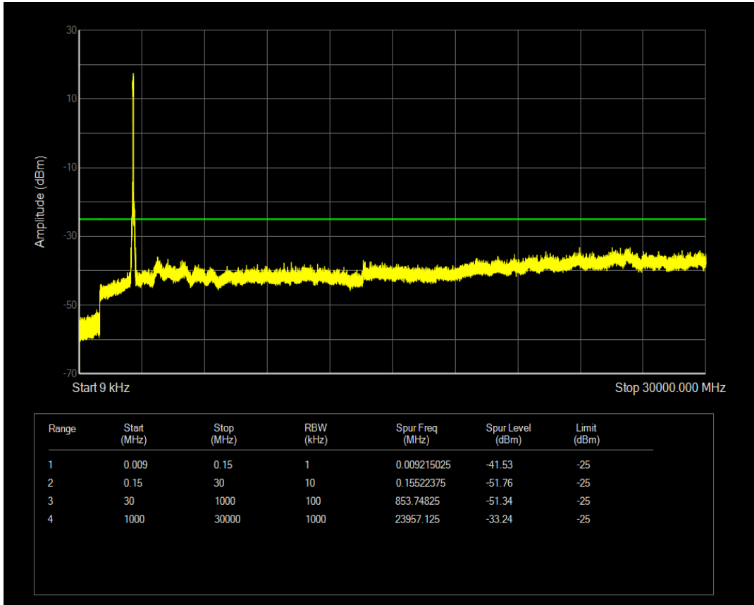
n41 SCS=15kHz DFT_QPSK BW=50MHz Channel=518601 RB=1@0
