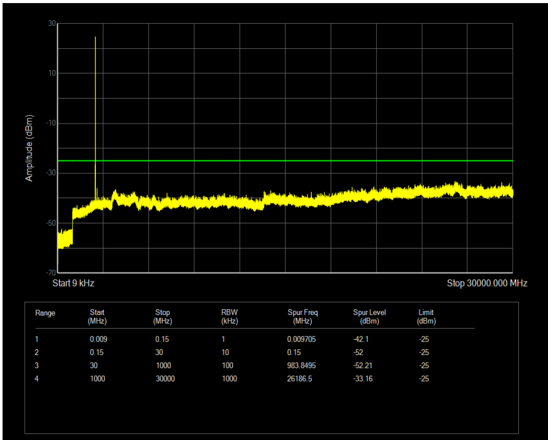
n41 SCS=15kHz DFT_QPSK BW=10MHz Channel=518601 RB=1@0
