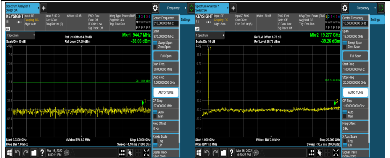
Band2-20MHz-QPSK-18900-1RB#0-Range1:30~1000MHz Band2-20MHz-QPSK-18900-1RB#0-Range2:1000~20000MHz
