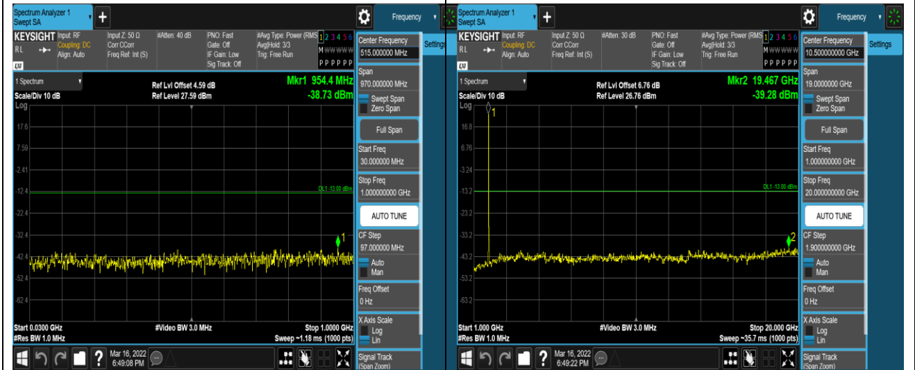
Band2-20MHz-QPSK-18900-1RB#0-Range1:30~1000MHz Band2-20MHz-QPSK-18900-1RB#0-Range2:1000~20000MHz
