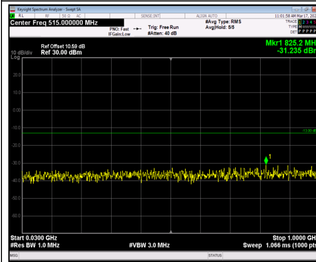
Band25-1.4MHz-16QAM-26365-1RB#0-Range1:30 ~1000MHz
