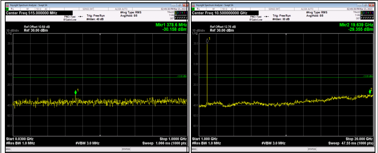
Band25-20MHz-QPSK-26140-1RB#0-Range1:30~1 000MHz
