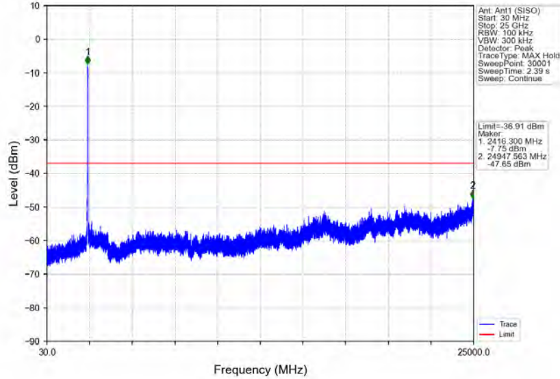
802.11n(HT40)_MCH_2437MHz_Ant1 (SISO)_NTNV
