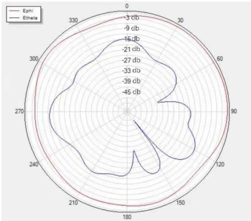
Theta=90 freq=2500MHz
