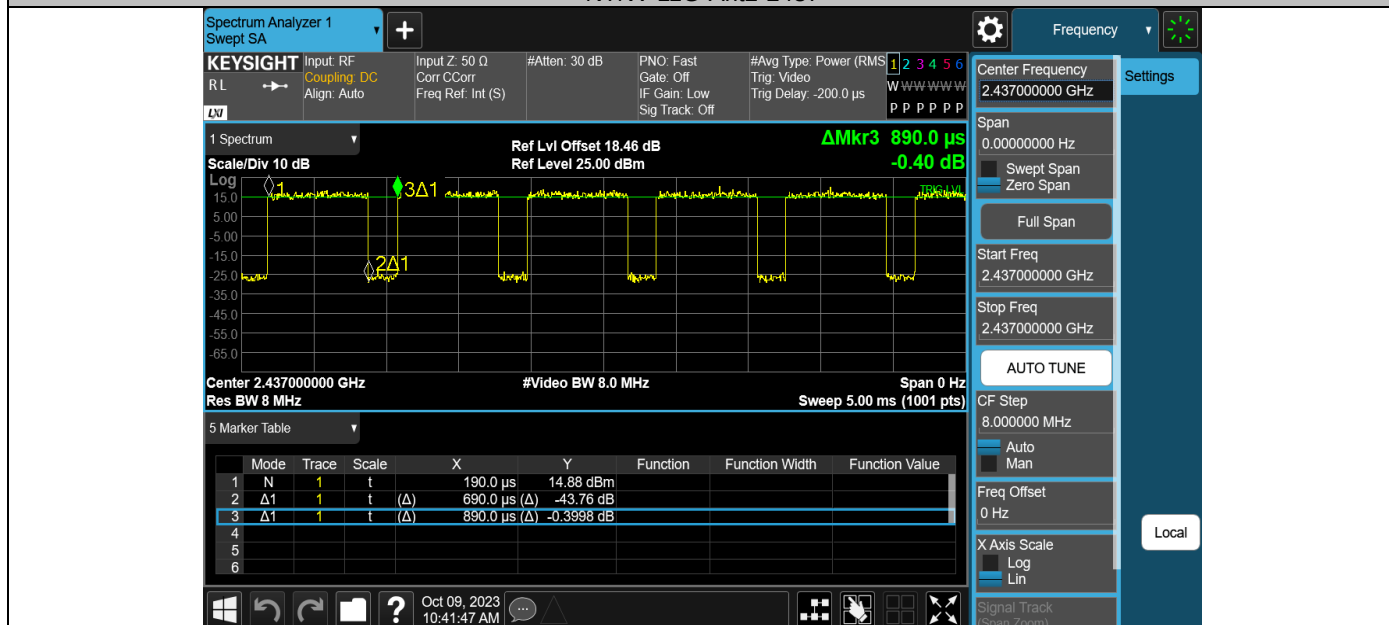
NTNV-11N20MIMO-Ant1-2437
