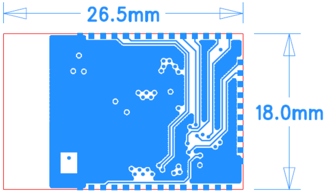
Inner Layer 3
