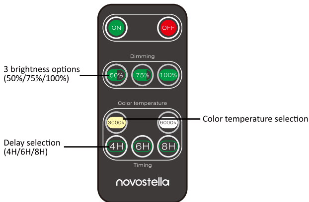
IR remote control
