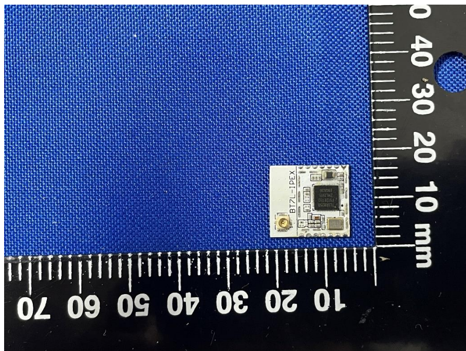
BLE MODULE UNCOVER TOP VIEW
