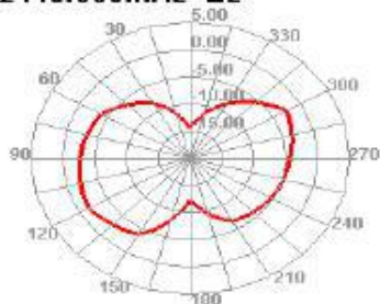
2440.000MHz E2
