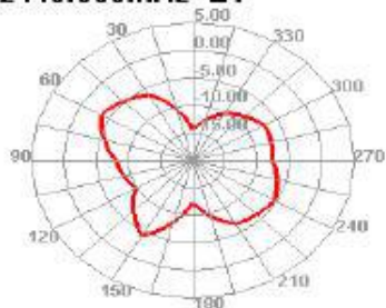
2440.000MHz E1
