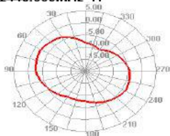
2440.000MHz E2
