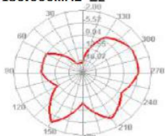
2480.000MHz E2
