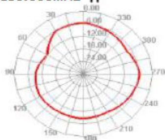
2480.000MHz H
