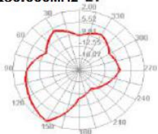
2480.000MHz E1
