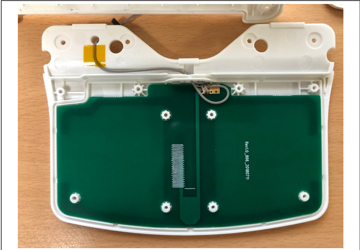
Antenna(UHF RFID)
