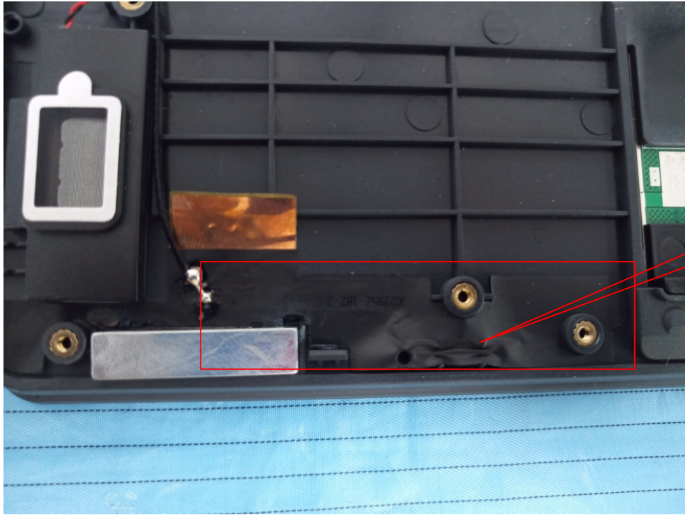
LTE Antenna
