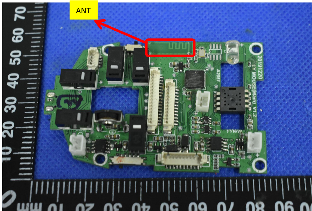
Antenna
