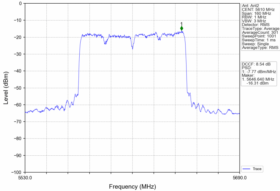
802.11ax(HEW80)_HCH_5610MHz_RU996_Left_MIMO_NTNV
