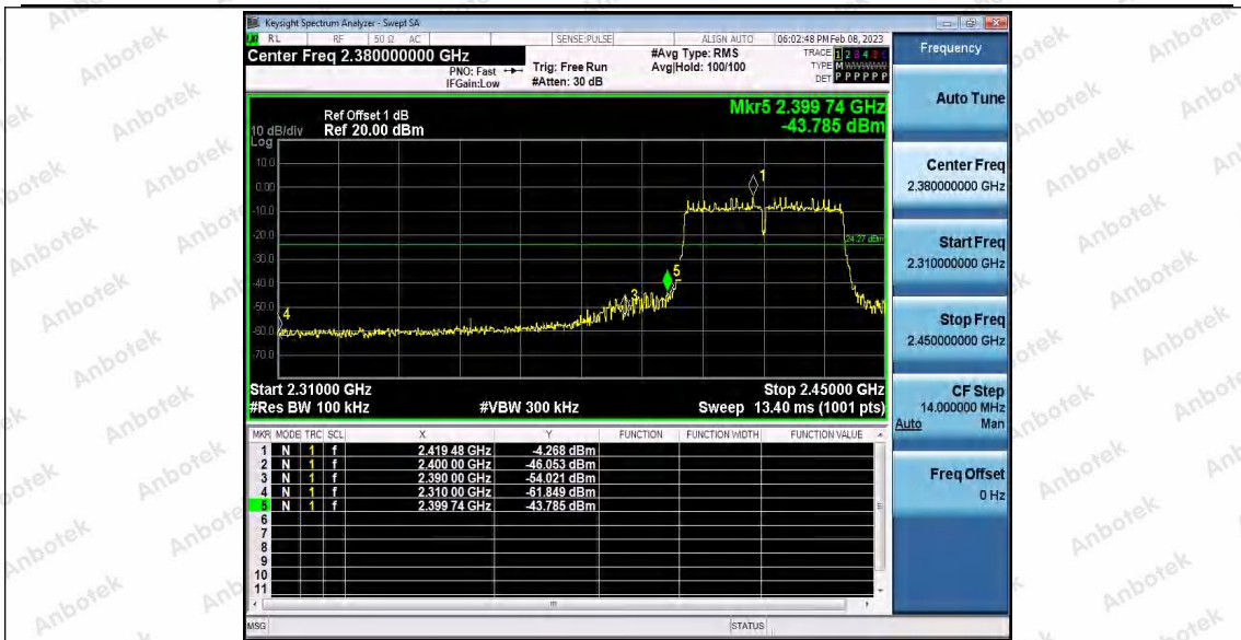
11N40_Ant2_Low_2422
