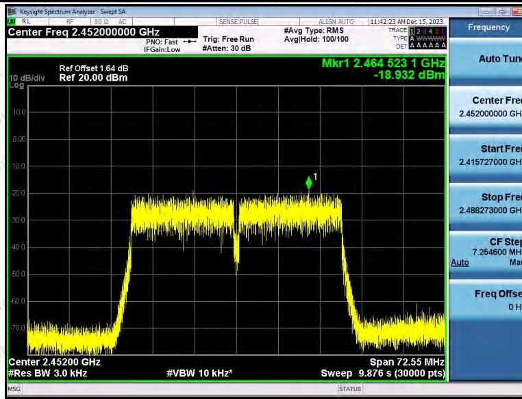
11N40SISO_Ant2_2452
