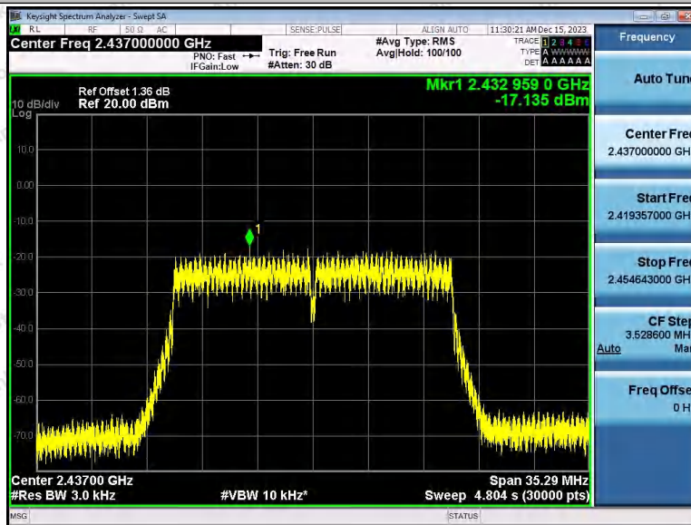
11N20SISO_Ant1_2437
