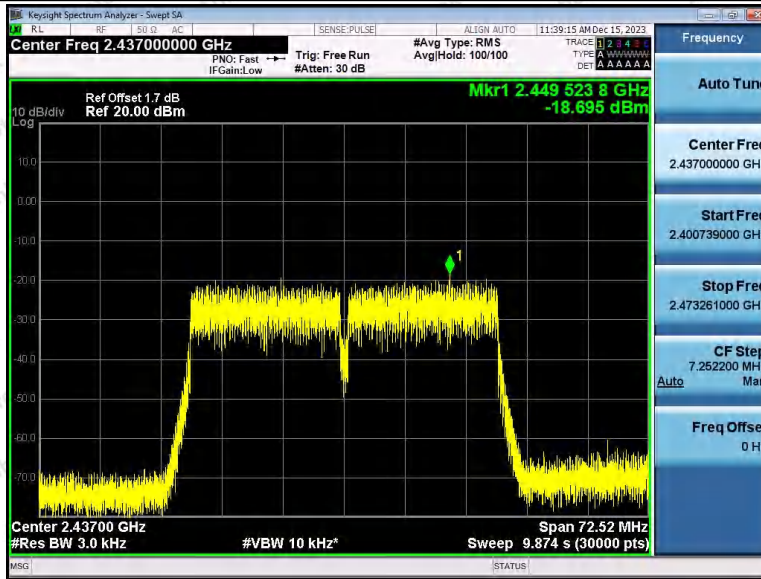
11N40SISO_Ant2_2437
