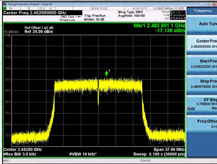
11AX20SISO_Ant2_2462
