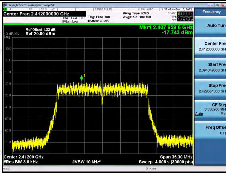
11N20SISO_Ant2_2412
