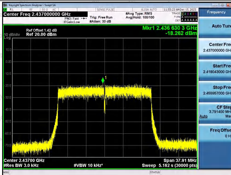
11AX20SISO_Ant2_2437
