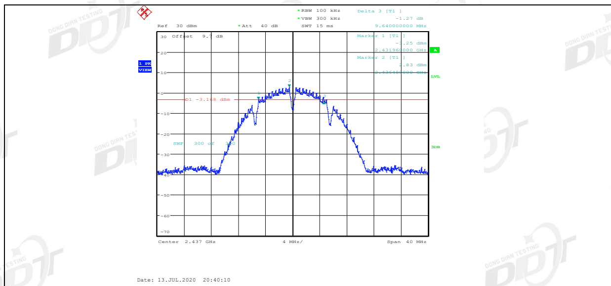
11B Ant2 2437
