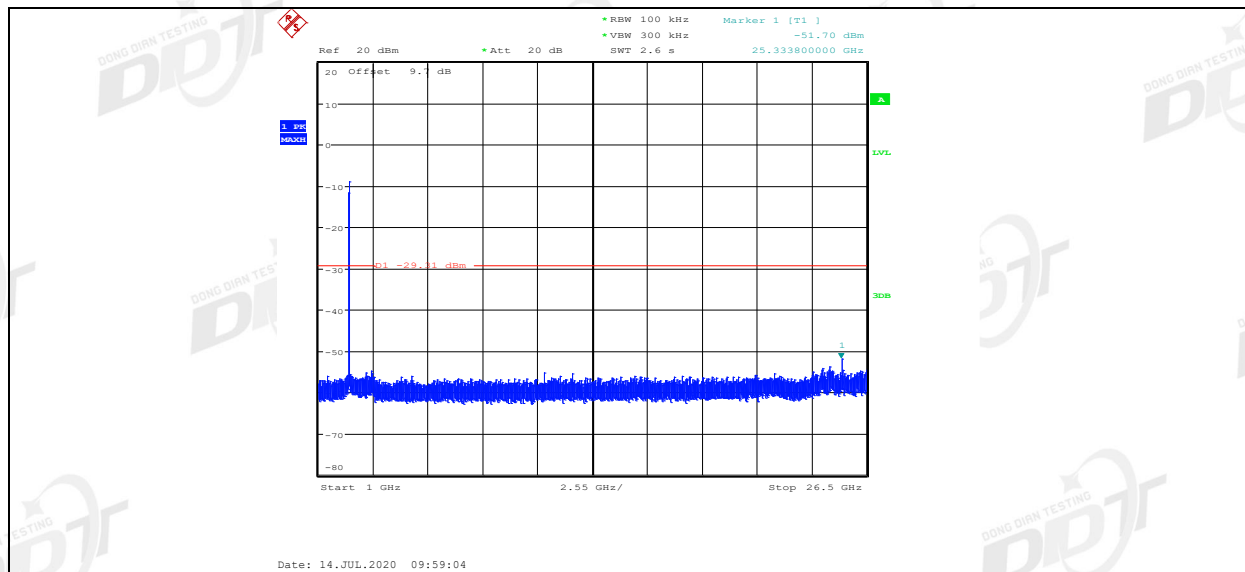
11N40MIMO_Ant2_2437_0-Reference
