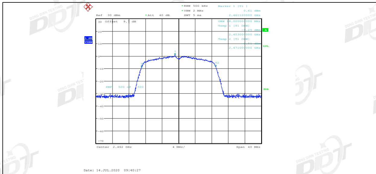
11N20MIMO Ant2 2462
