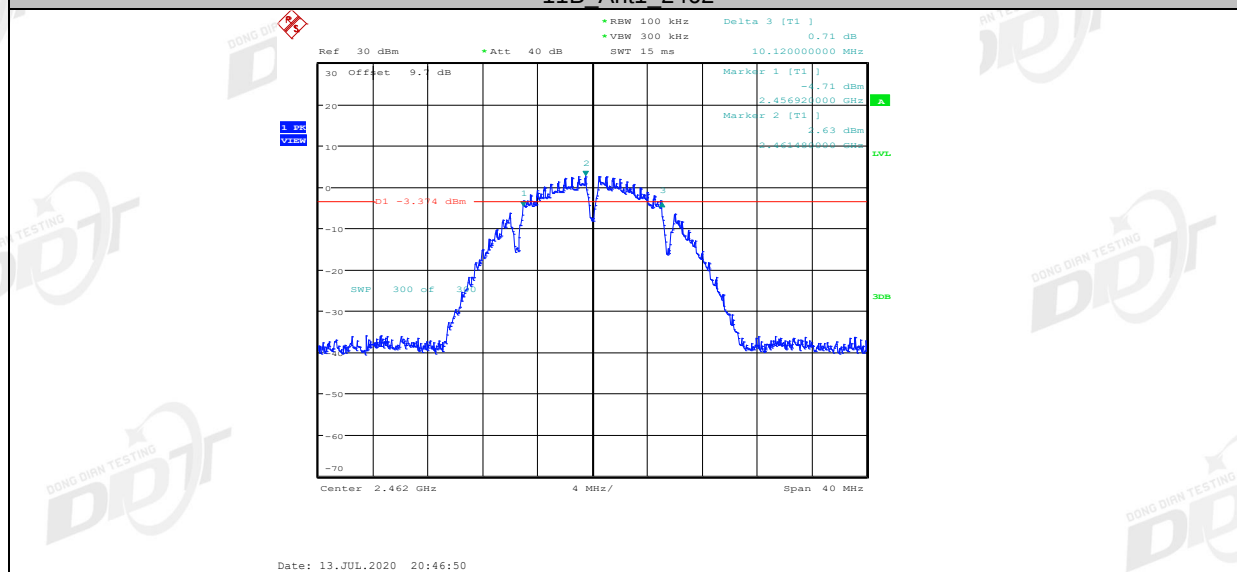
11B Ant2 2462
