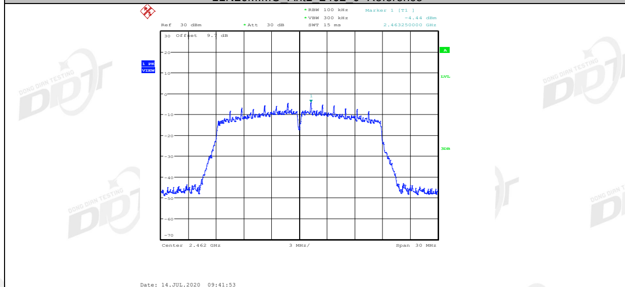
11N20MIMO_Ant1_2462_30-1000
