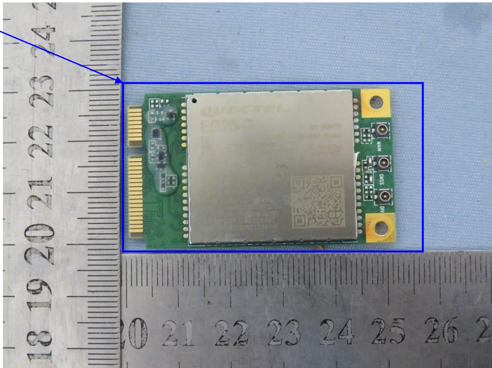
LTE Module
