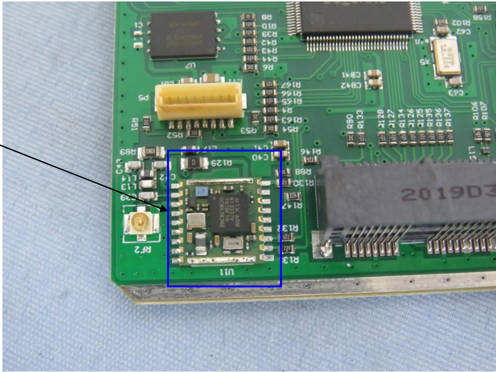
GPS Module
