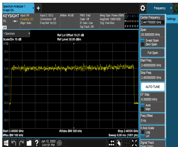
3DH5_Ant1_Hop
