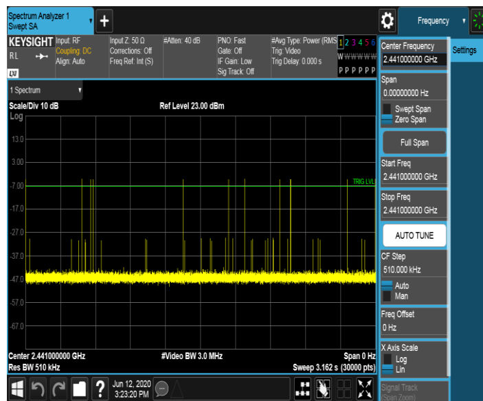
DH3_Ant1_Hop
