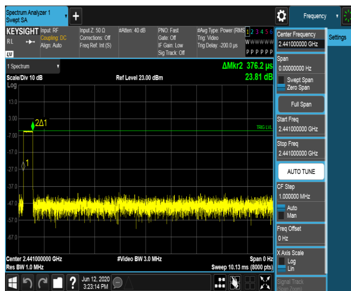
DH1_Ant1_Hop
