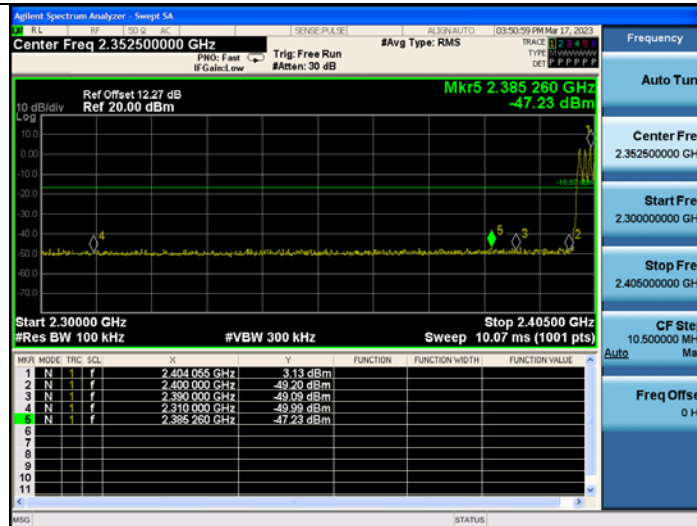
DH5 Left High Hop 2480
