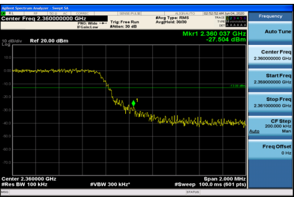
HCH_QPSK_25RB#0
