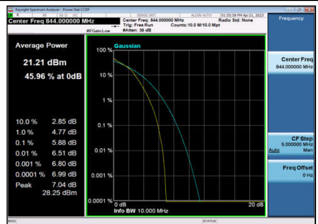
FDD05_HighRange_10MHz_844_fullIRB_high_Q16
