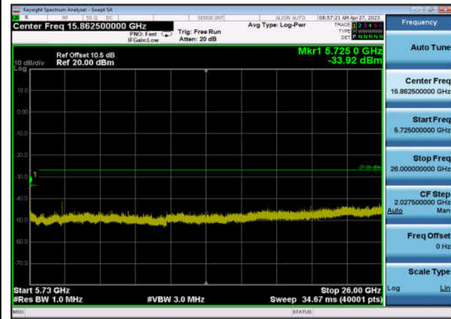
U-NII-2c ,Plot 3,5725MHz~26000MHz-802 .11ac(20MHz),5600MHz,Ant1
