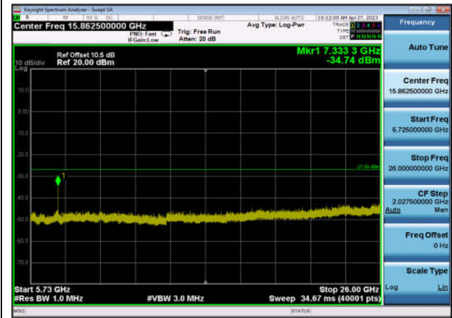
U-NII-2c ,Plot 3,5725MHz~26000MHz-802 .11ac(20MHz),5700MHz,Ant1
