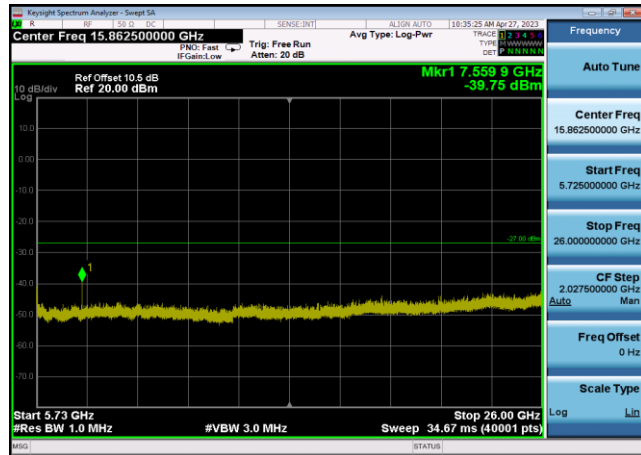
U-NII-2c ,Plot 3,5725MHz~26000MHz-802 .11ac(80MHz),5610MHz,Ant1
