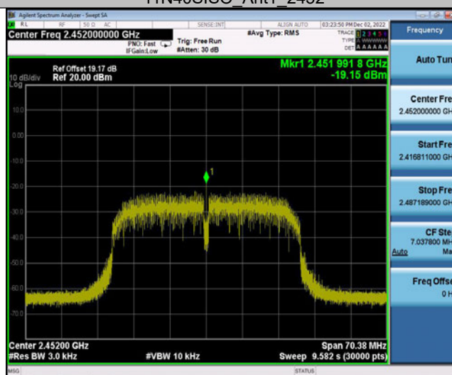
11N40SISO Ant1 2452
