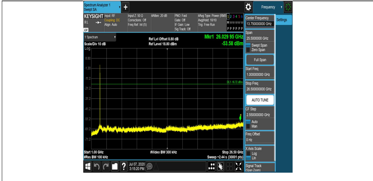
11B_Ant1_2462_0~Reference
