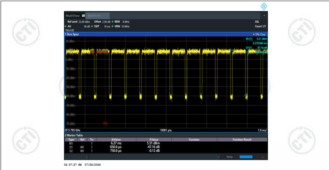
11N40SISO_Ant2_5795
