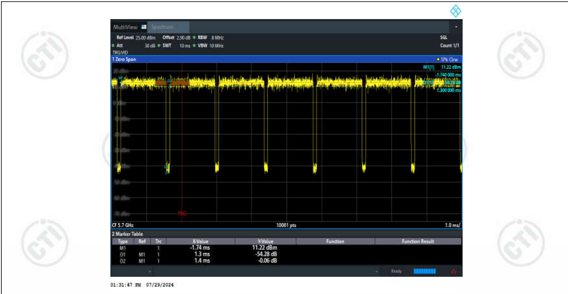
11N20SISO_Ant2_5700
