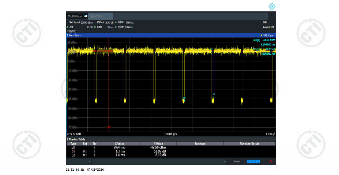
11N20SISO_Ant2_5220
