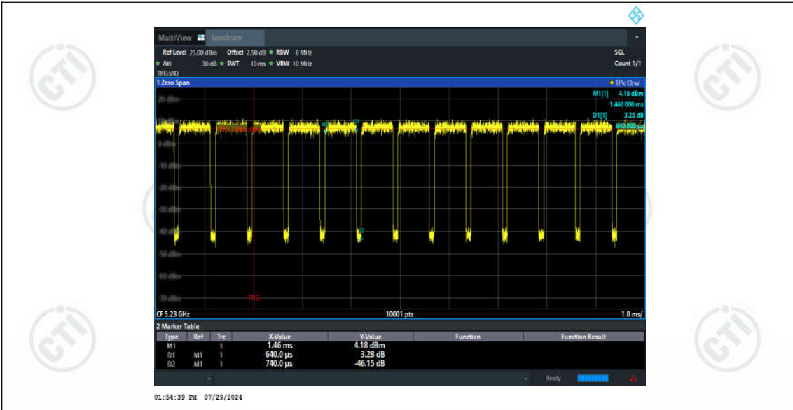
11N40SISO_Ant2_5230
