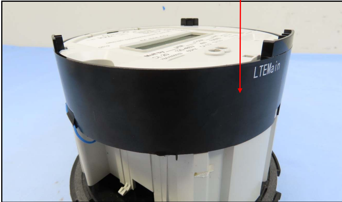
LTE antenna
