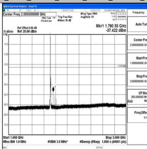
Band66 5MHz 16QAM 131997 1RB#0 1000~3000 1000~3000
