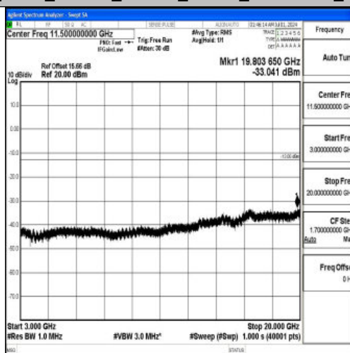
Band66 5MHz 16QAM 131997 1RB#0 3000~20000 3000~20000
