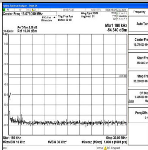
Band66 20MHz QPSK 132572 1RB#0 0.15~30 0.15~30
