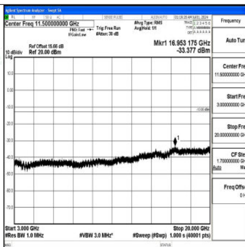
Band66 3MHz QPSK 131987 1RB#0 3000~20000 3000~20000
