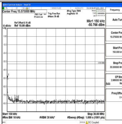
Band66 3MHz 16QAM 131987 1RB#0 0.15~30 0.15~30
