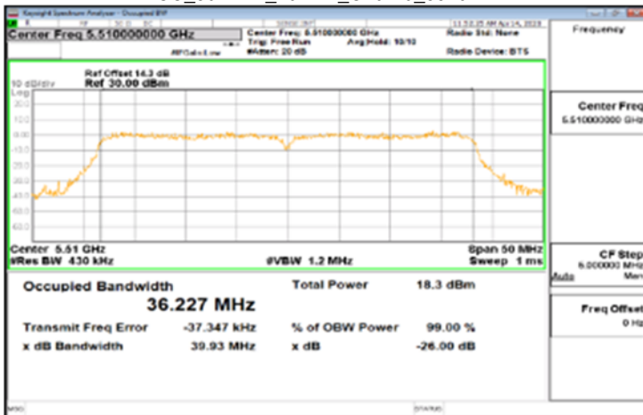
FCC 802.11n_40MHz_Chain0_5510MHz
