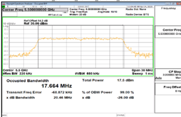
FCC 802.11n_20MHz_Chain0_5500MHz
