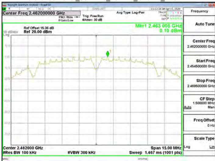
Reference Level_802.11b_20MHz_Chain1_2462MHz
