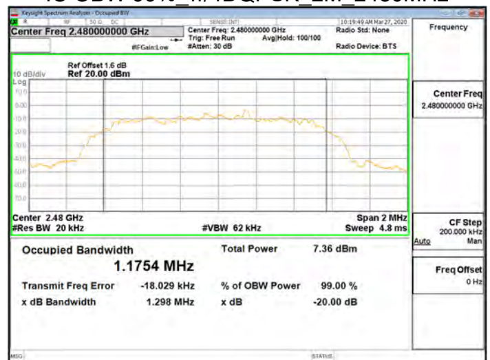
IC OBW 99% π/4DQPSK 2M 2480MHz
