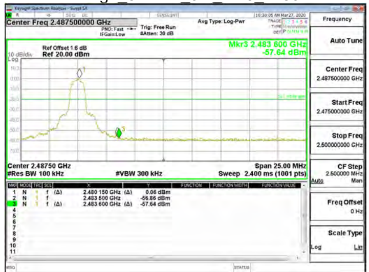
Band Edge 8DPSK 3M DH5 2480MHz
