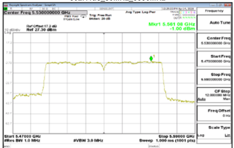
802.11ac_80MHz_5530MHz
