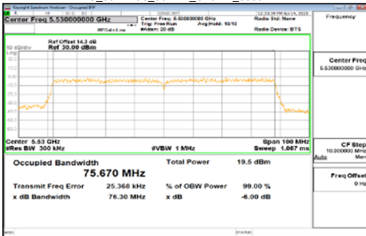
IC_802.11ac_80MHz_Chain1_5530MHz
