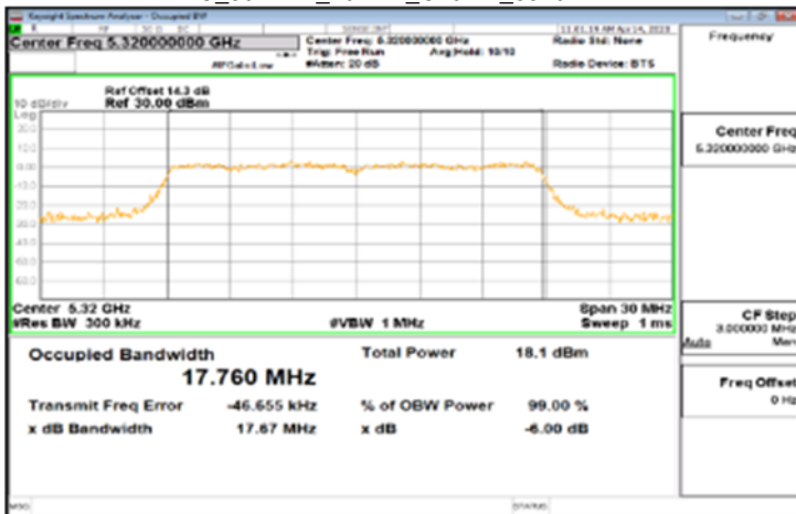
IC_802.11n_20MHz_Chain1_5320MHz
