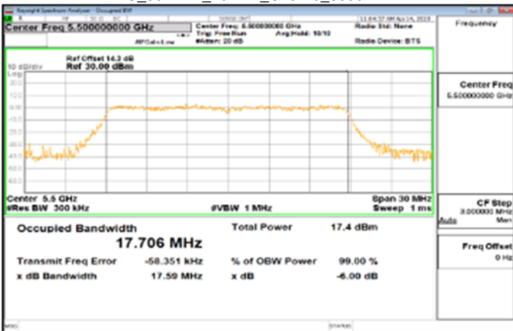
IC_802.11n_20MHz_Chain0_5500MHz
