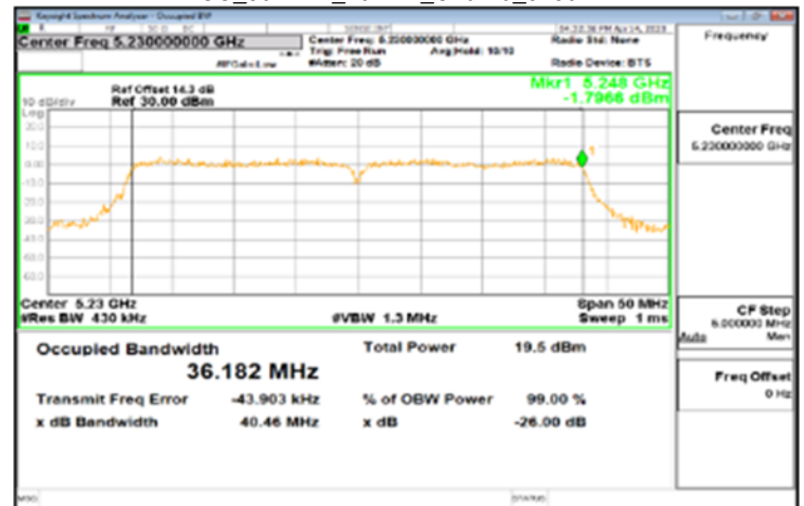
FCC 802.11n_40MHz_Chain0_5230MHz
