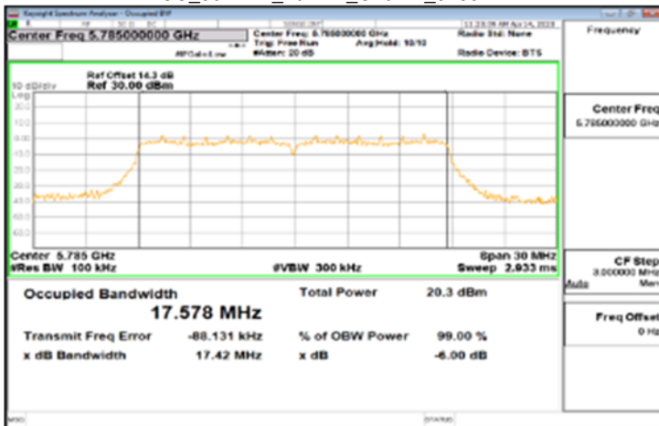
FCC 802.11n_20MHz_Chain1_5785MHz
