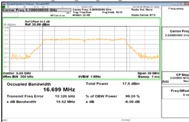
IC_802.11a_20MHz_Chain1_5580MHz
