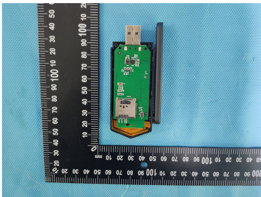
WCDMA/LTE ANT.
