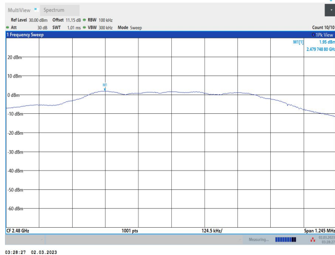
BLE 1M_Ant1_2480
