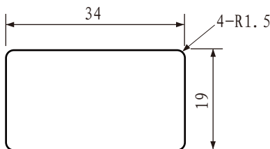
结构尺寸图
