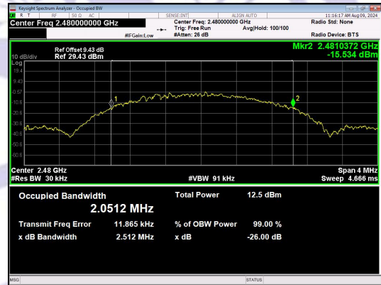
BLE 2M_Channel 39
