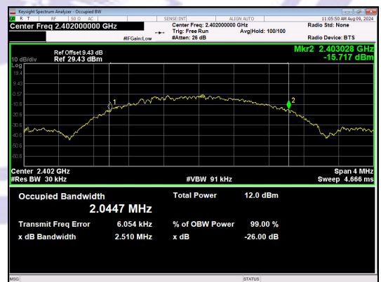
BLE 2M_Channel 0
