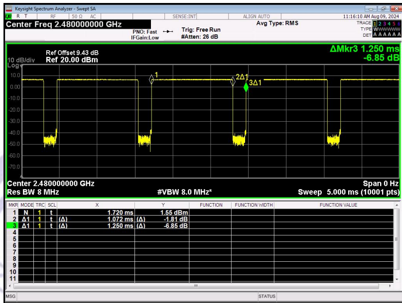
BLE 2M_Channel 39
