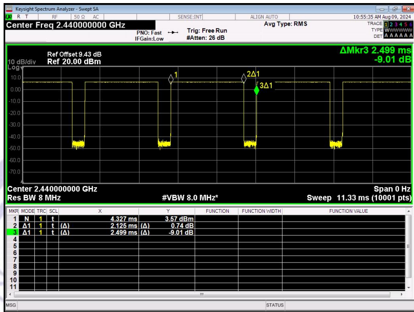
BLE 1M_Channel 19
