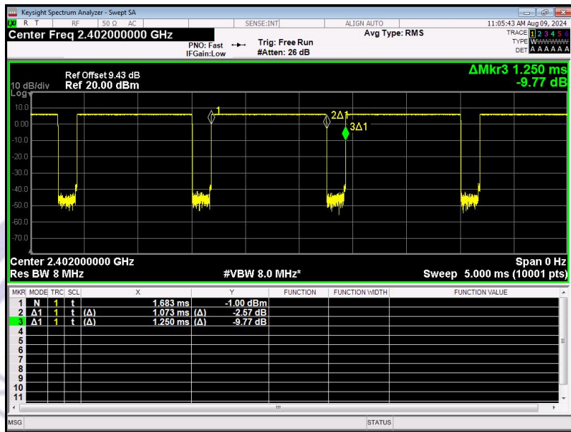
BLE 2M_Channel 0
