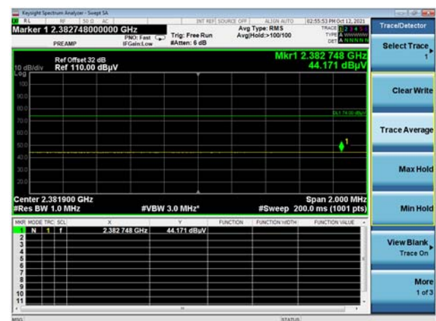
GFSK 1M LOW CHANNEL, AV
