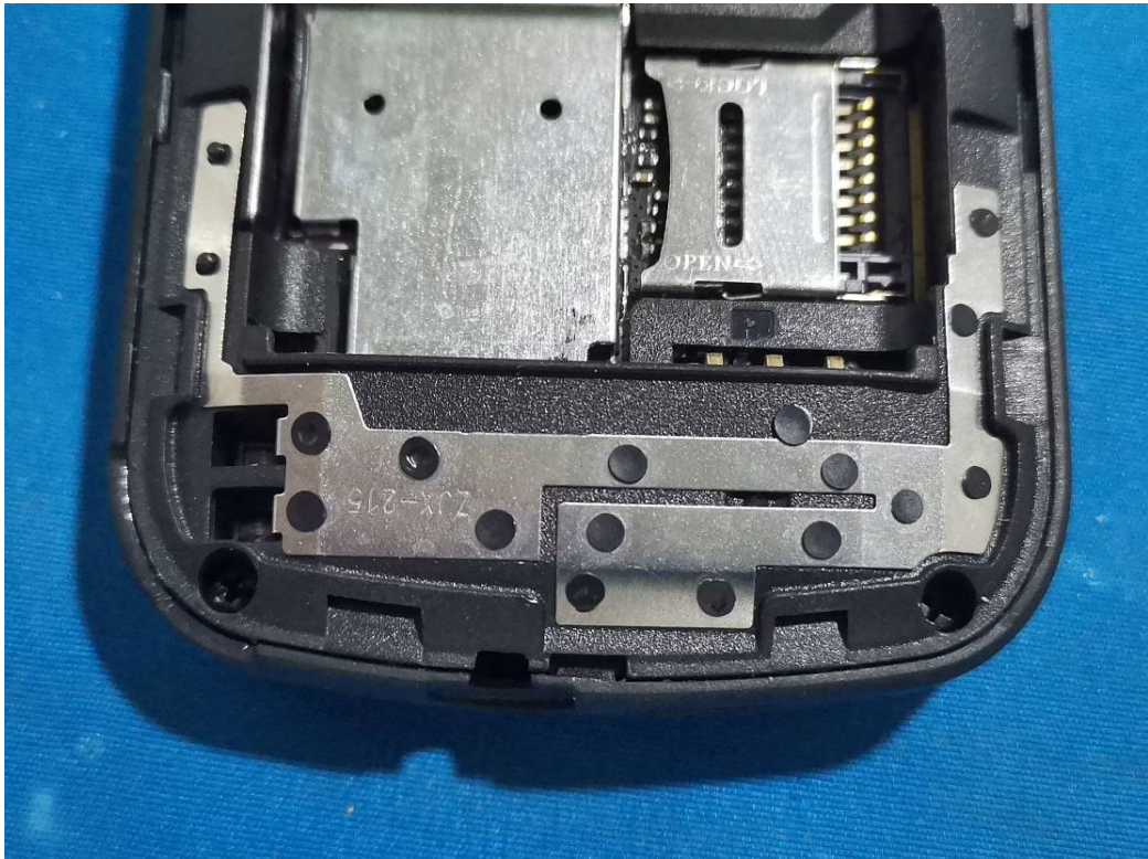
GSM ANT
