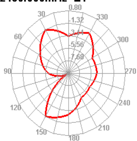
2480.000MHz E1
