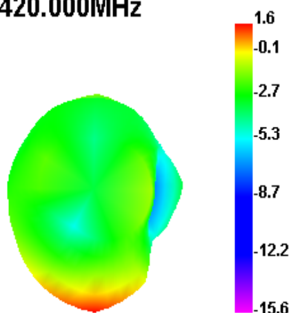
2420.000MHz E1
