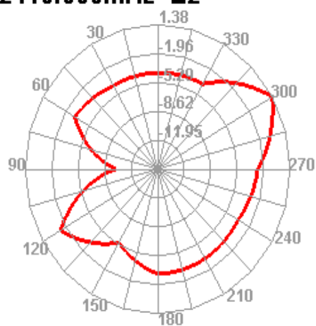
2420.000MHz H
