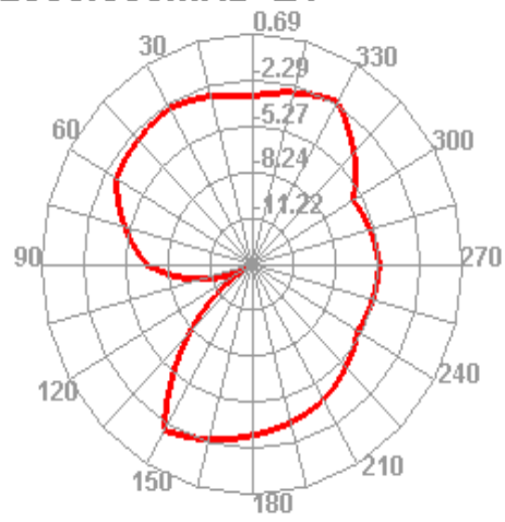
2500.000MHz E1
