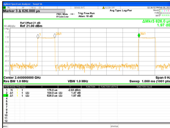
Duty Cycle @ BLE 2M Mode Ch 19
