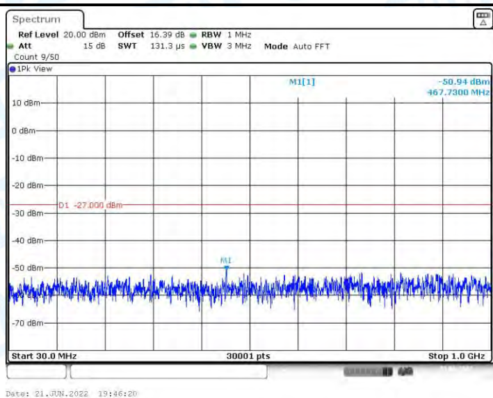
11N20MIMO_Ant2_5300_30~1000
