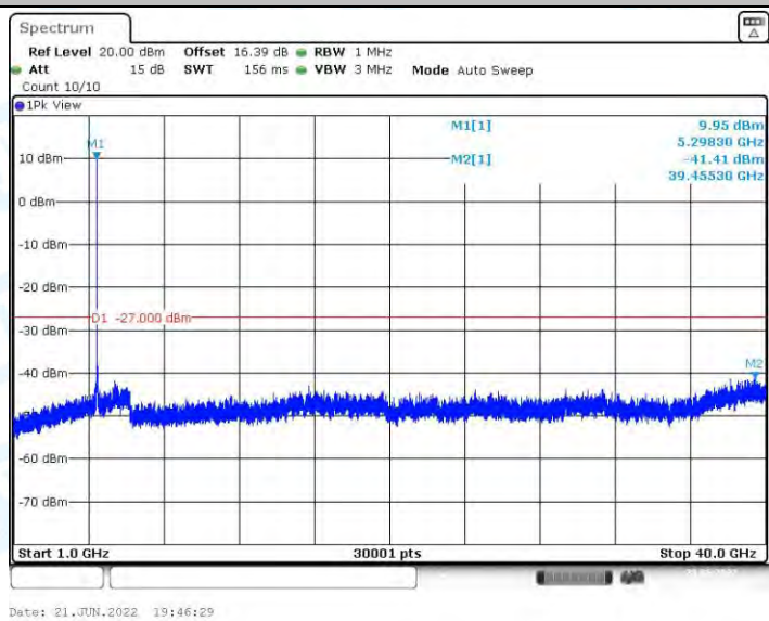
11N20MIMO_Ant2_5300_1000~40000
