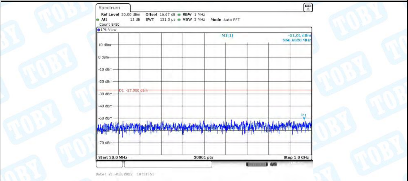
11A_Ant2_5500_30~1000
