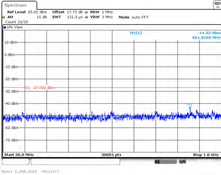
11A-Ant1-5745-30~1000-PASS
