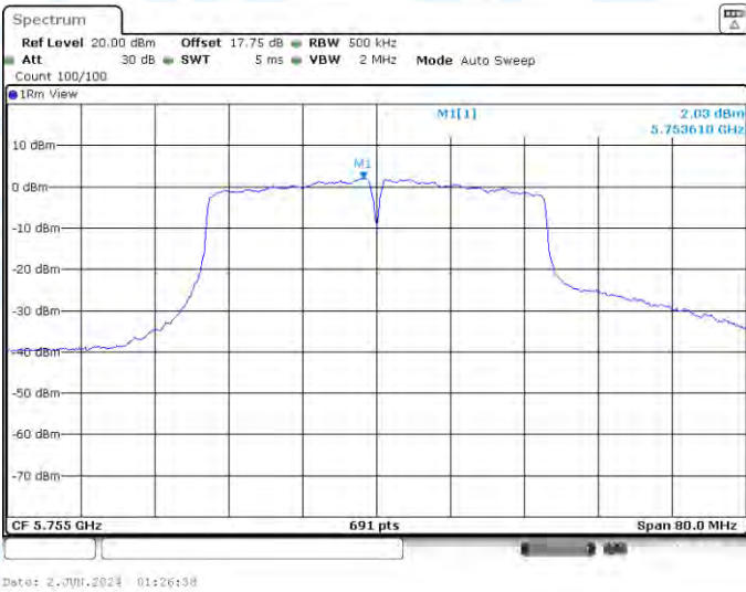
11N40-CDD-Ant2-5755-PASS
