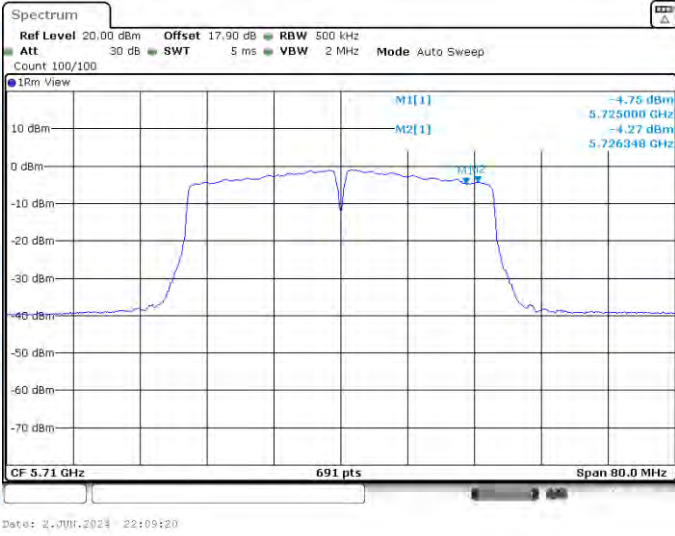
11N40-CDD-Ant1-5710_UNII-3-PASS
