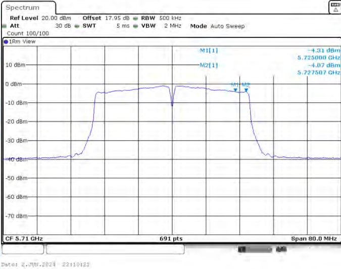
11N40-CDD-Ant3-5710_UNII-3-PASS
